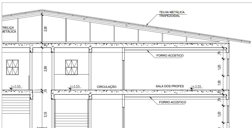
Figura 01: Projeto Especificação telhado
