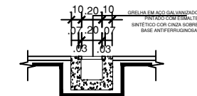
CORTE - CANALETA E GRELHA METÁLICA ESC.: 1/50
