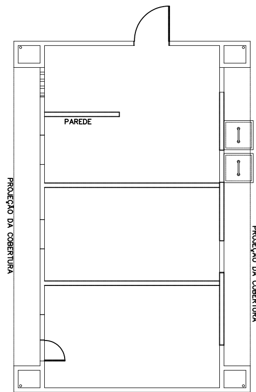
PLANTA DE DEMOLIÇÃO E CONSTRUÇÃO ESC.: 1/125
