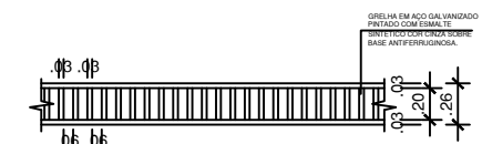
VISTA SUPERIOR - CANALETA E GRELHA METÁLICA ESC.: 1/50
